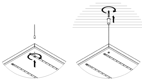
Рисунок 7 — Подвесной монтаж.
